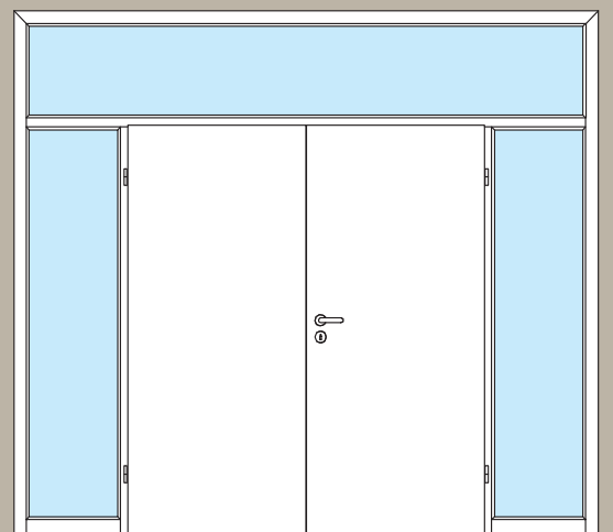
2-flügelig, 2 Seitenteile, 1 Oberlicht
