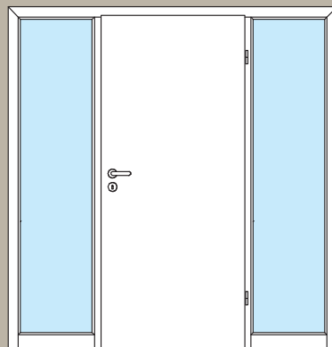
1-flügelig, 2 Seitenteile
