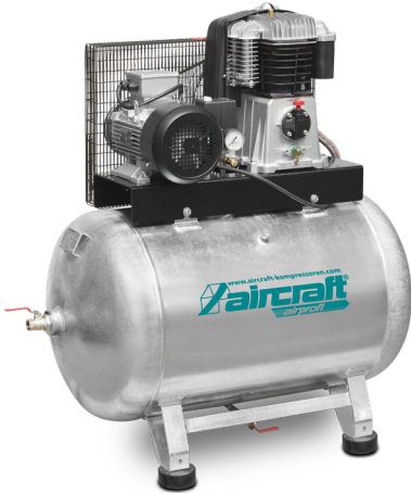
AIRPROFI 853/270/10 H 2-Zylinder-Kompressor auf 270 Liter Druckluft-Behälter
