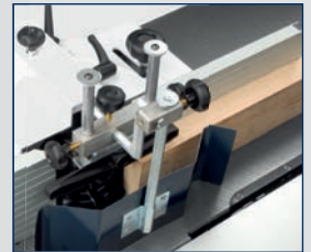
Der Standard-Frässchutz ist für maximale Sicherheit. Höhenverstellbare Führungsschiene und Schutzblech
