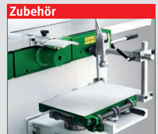
Langlochbohrereinrichtung Wescott 0 - 16 mm
