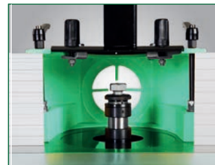
Frässpindel mit 80 mm Nutzlänge und 30 mm Durchmesser
