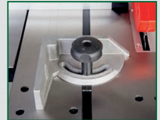
Stufenlos verstellbarer Winkelanschlag von -45° bis +45°
