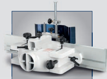
Integrierter Absauganschluss sorgt für freie Sicht beim Fräsen. Frässchutz für maximale Sicherheit mit höhenverstellbarer Schutzschiene und einem Schutzblech
