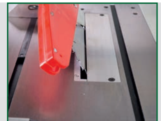
Sägeblattschwenkung von 90° bis -45° nach links
