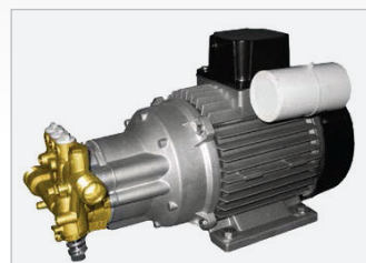
Elektrische Drei-Kolben-Axialpumpe mit Messingkopf Induktionsmotor mit Motorschutzschalter
