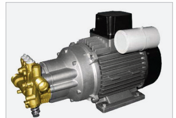
Elektrische Drei-Kolben-Axialpumpe mit Messingkopf Induktionsmotor mit Motorschutzschalter
